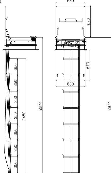
측면도
