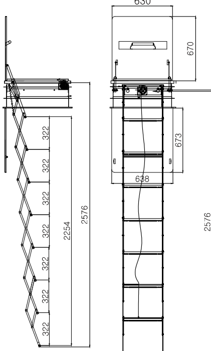
측면도
