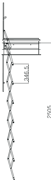
측면도
